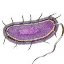
Клетка бактерии
